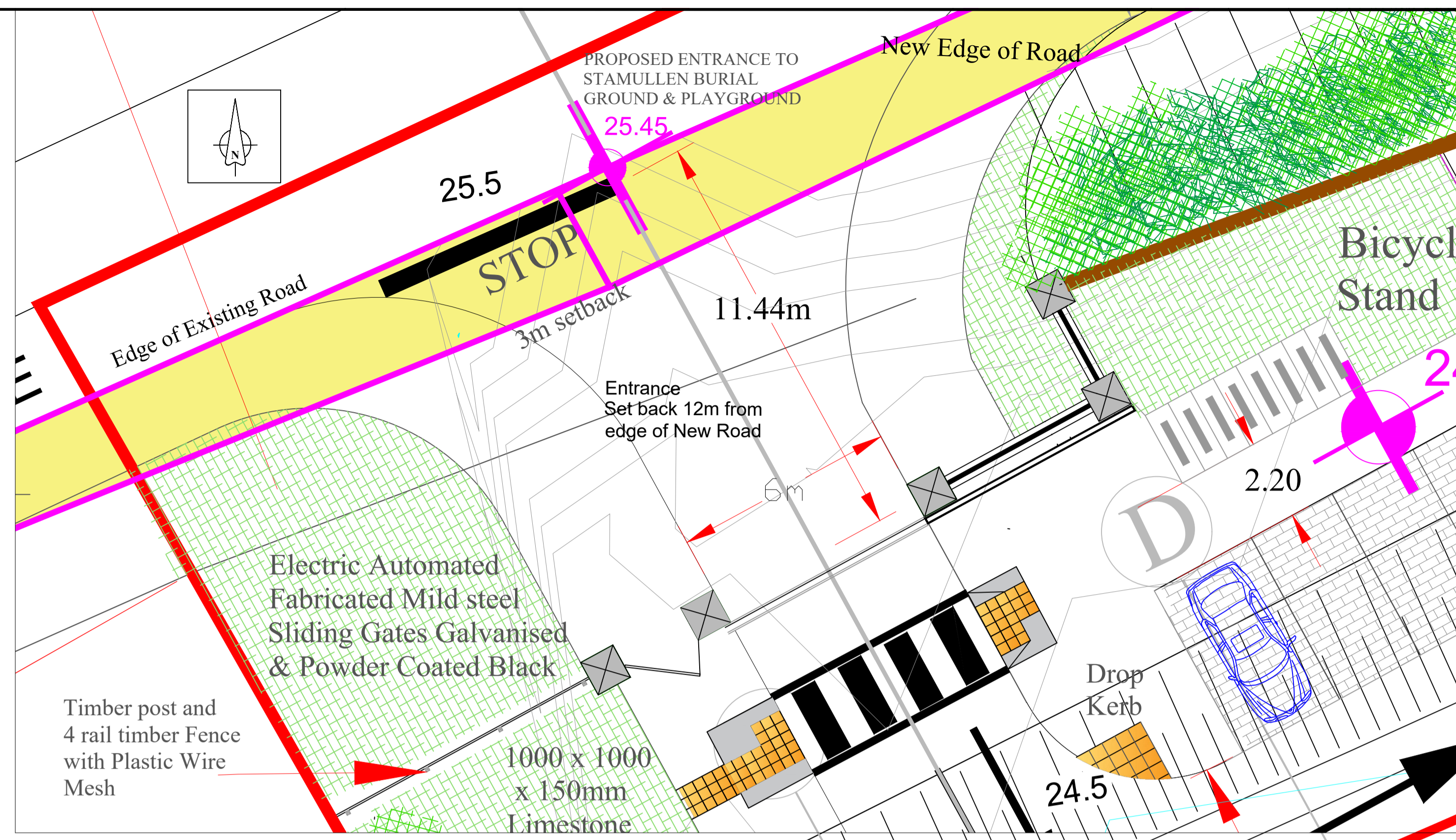
Entrance Plan Scale: 1:200
